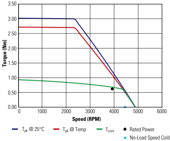
TBM(S)-7615-A 48 Vdc – 6 step
